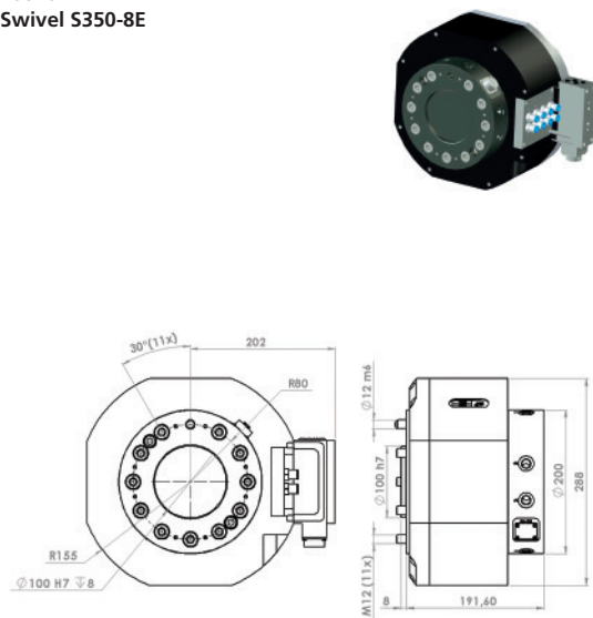
P0610 Swivel S350-8E
